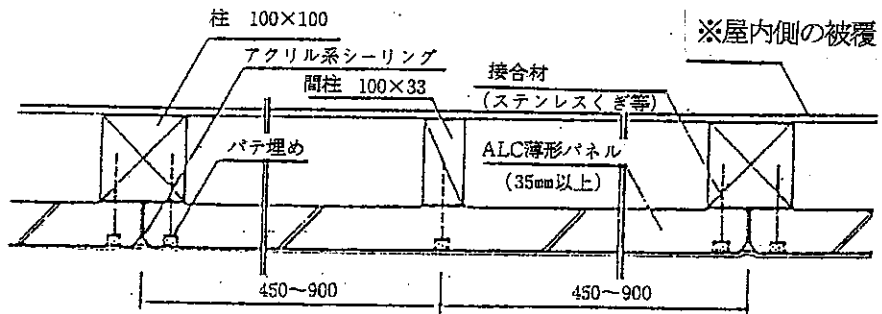
A-A 断面図
