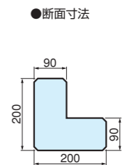
●断面寸法
